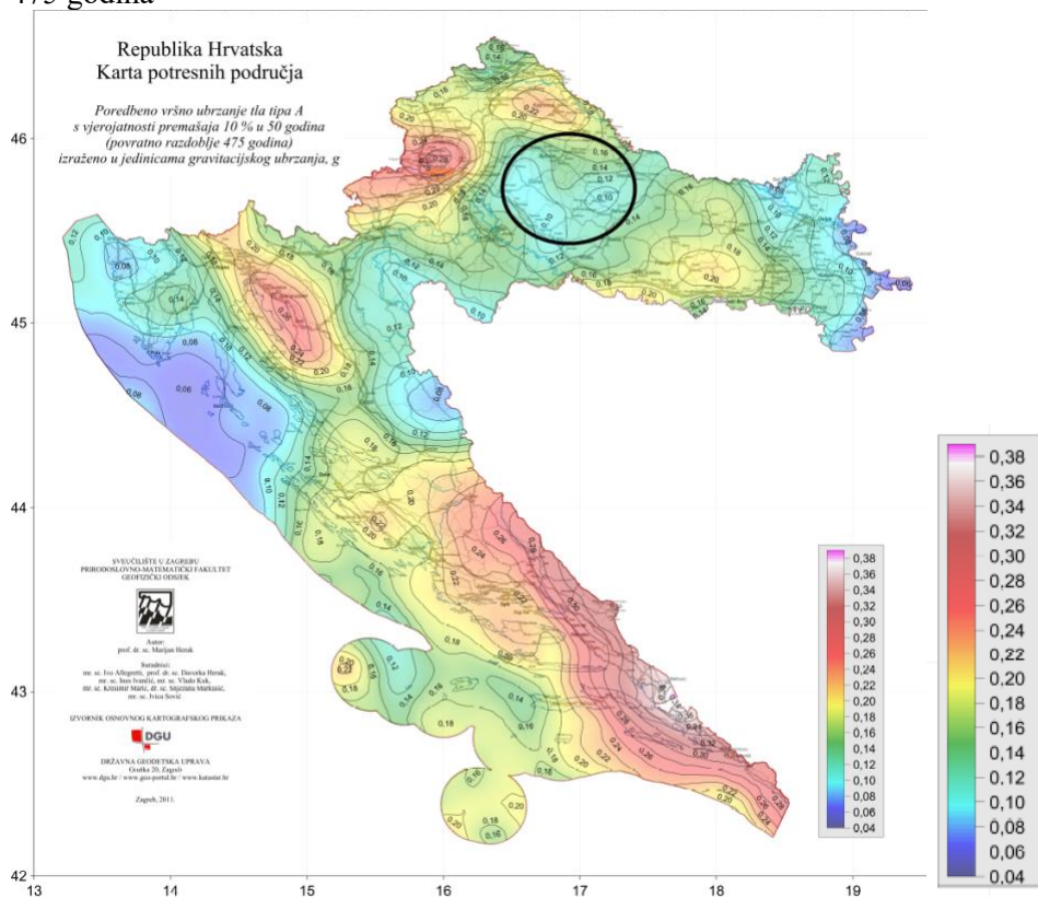
Slika 6: Izvod iz Karte potresnih područja u RH; Poredbeno vršno ubrzanje tla tipa A, povratno razdoblje 475 godina
